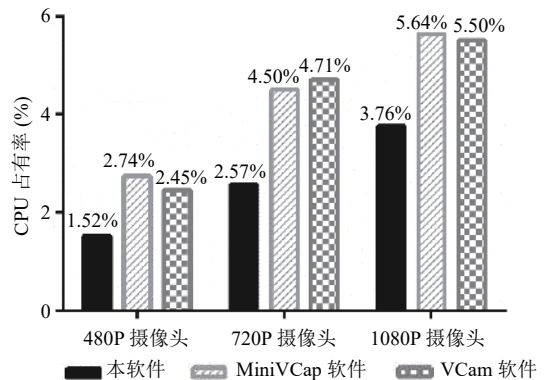
图 9 CPU 占有率测试结果
