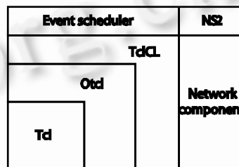
图 1 NS2 分裂对象模型架构图
