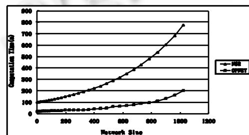
图7 CPU计算时间(丢包率=0.1)
