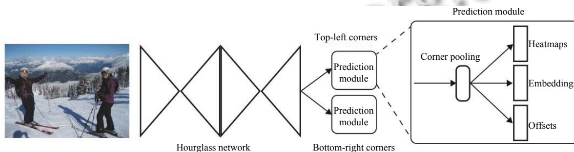
图 1 CornerNet 流程图 [4]
